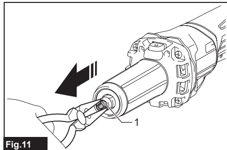
► 1. Collet cone
